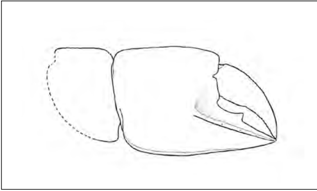
Fig. 2 - Calliaxina altavillensis sp. nov., ricostruzione della chela / reconstruction of the chela.
